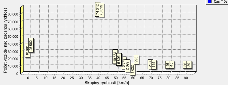
Graf rychlosti osobních, nákladních vozidel a souprav před zařízením v časech T 0s a T-5s za období od 01.03.25 00:00 do 31.03.25 23:59
