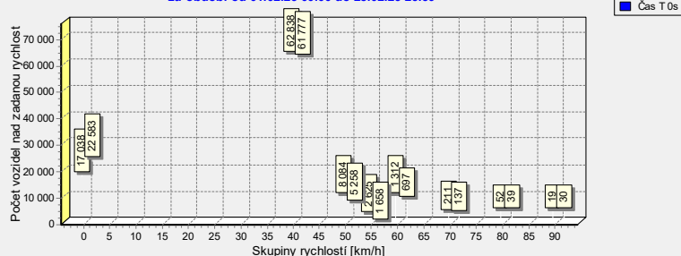
Graf rychlosti osobních, nákladních vozidel a souprav před zařízením v časech T 0s a T-5s za období od 01.02.25 00:00 do 28.02.25 23:59
